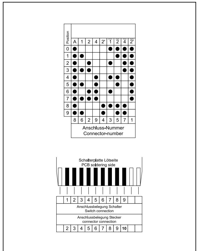
Code 140 BCD + 2 inputs
